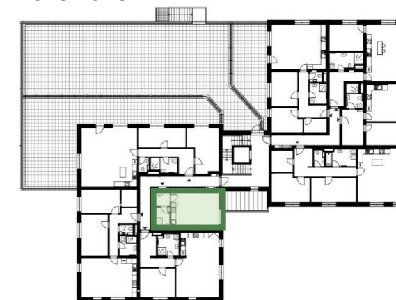
PŮDORYS PODLAŽÍ
